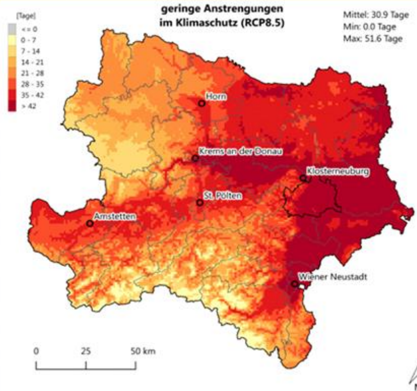
Zukünftiges Klima (2071-2100)
