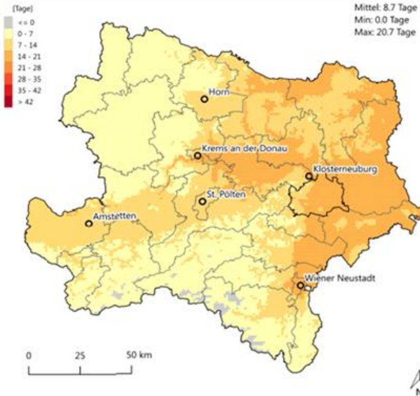
Aktuelles Klima (1981-2010)
